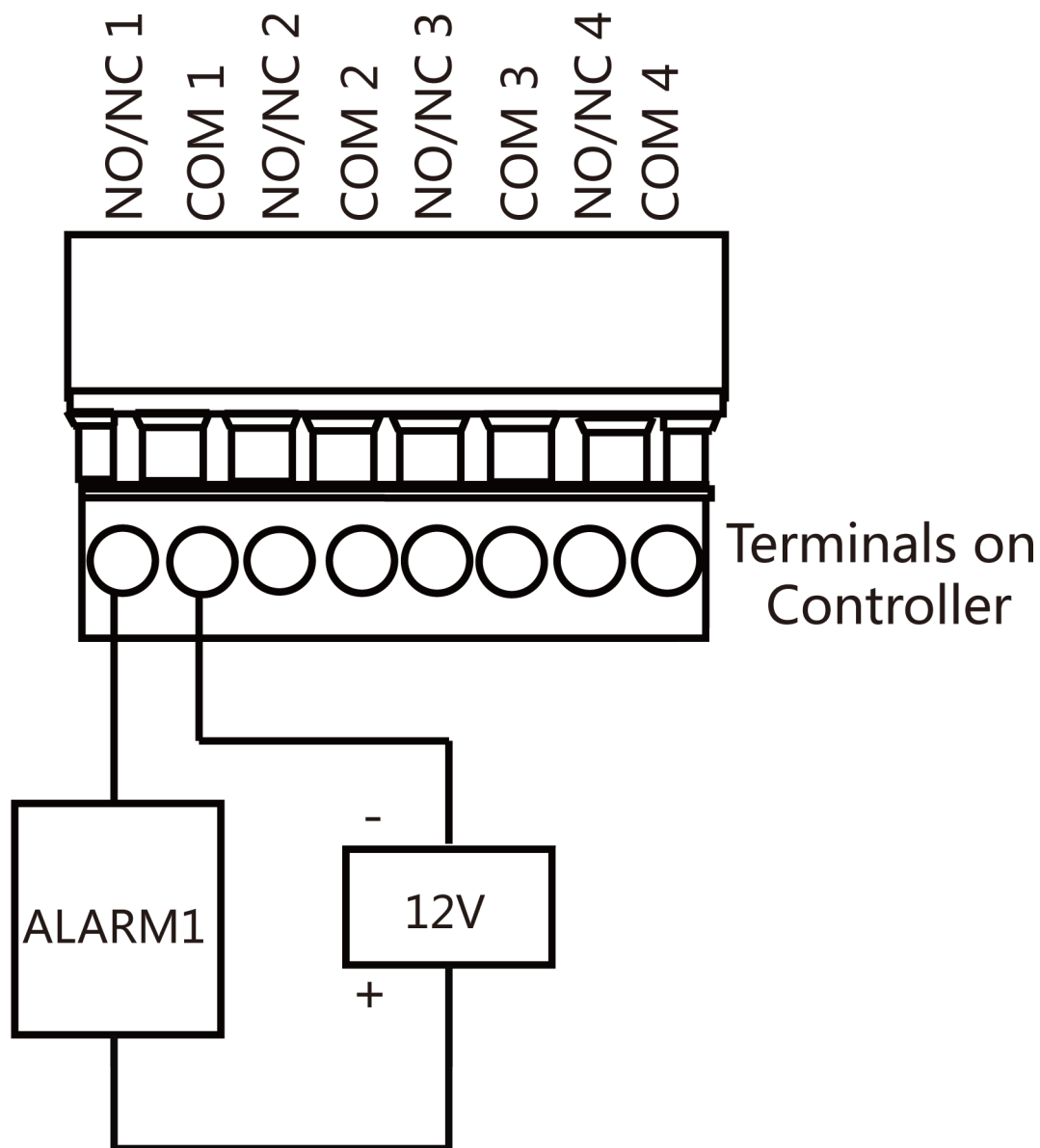
Рисунок 5-8. Подключение внешнего тревожного устройства
