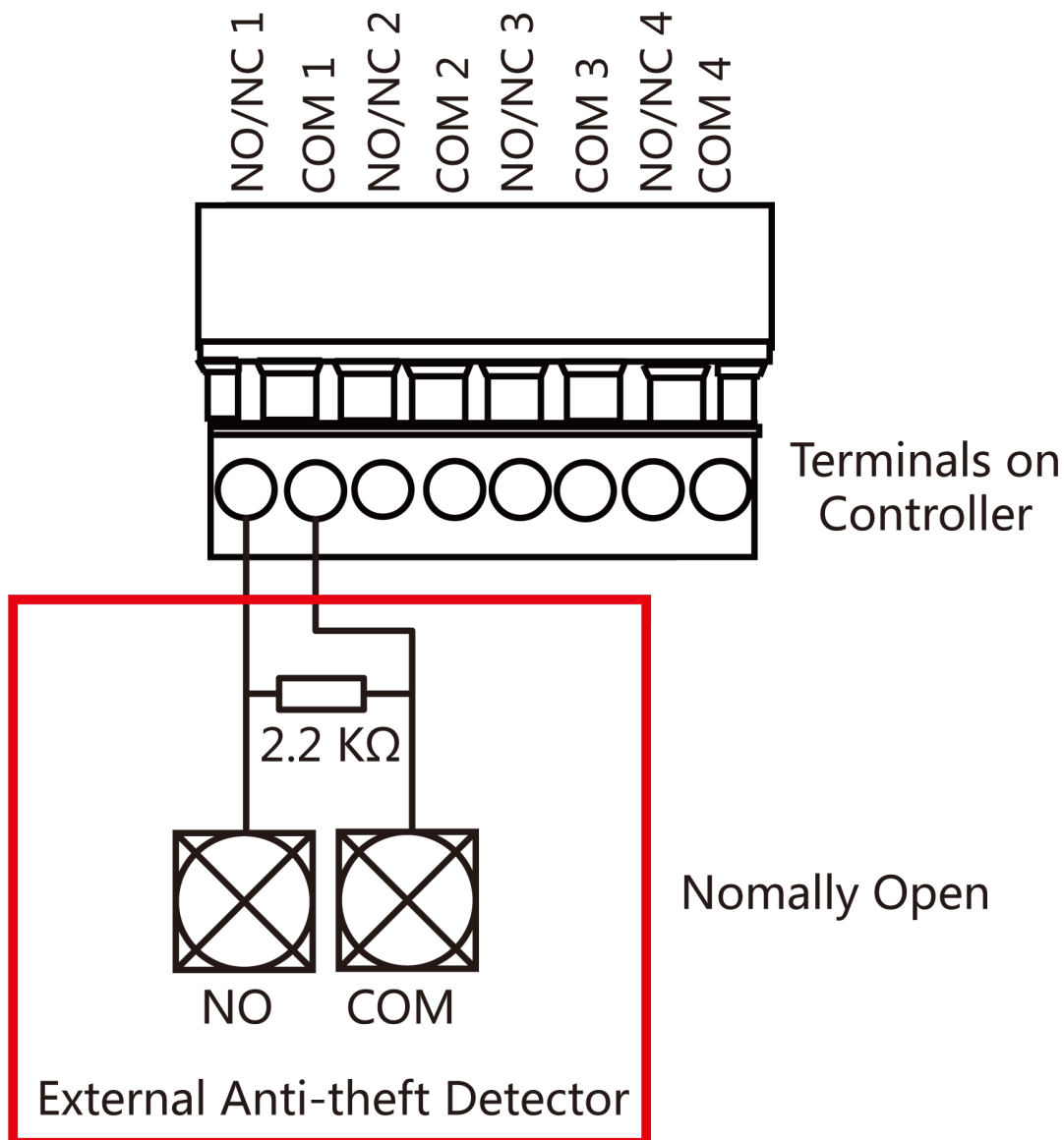
Рисунок 5-12. Подключение NO
