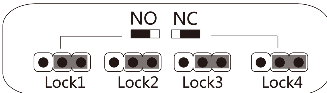
Рисунок 6-4. Состояние NC
