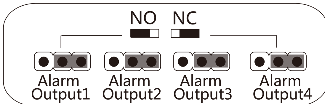
Рисунок 6-6. Состояние NC
