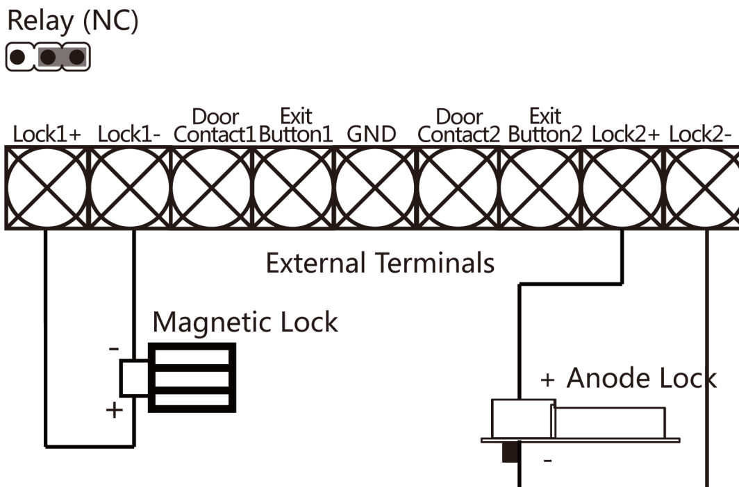
Рисунок 5-7. Схема подключения анодного замка
